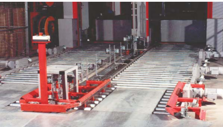
Winkelübergabe bei einer Bauhöhe von 80mm durch Hub-Staukettenförderer Angle transfer with pneumatic raisable buffer chain conveyor and a height of 80mm
