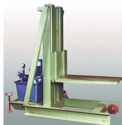
Verfahrbare Spezial-Hebevorrichtung Mobile special lifting installation
