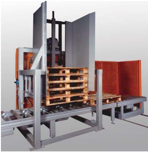
Palettenspender Serie 915 Pallet dispenser serie 915
